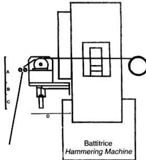
Applicazione sulla battitrice Application on hammering machine
